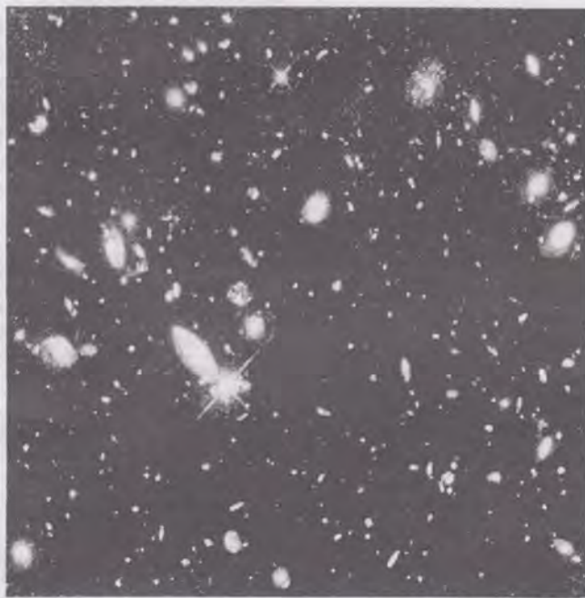
Galaxii îndepărtate, privite prin Telescopul Spațial Hubble (TSH). În această imagine pot fi văzute aproximativ 1500 de galaxii. Prin înmulțirea imaginii pentru a acoperi cerul întreg, se obține un total de 10 miliarde de galaxii care pot fi observate prin TSH.
