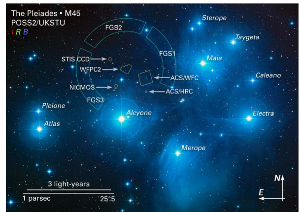
Fig. 5. Pleiadele
