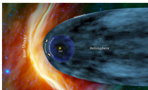
Fig. 3. Soarele – Termosfera – Heliosfera
