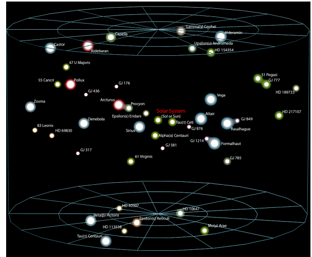
Fig. 4. Stele vecine Soarelui
