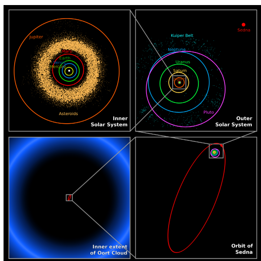
Fig. 2. Orbite – Norul lui Oort – Sedna
