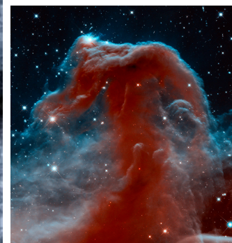
Fig. 9. Nebuloasa Cap-de-Cal
