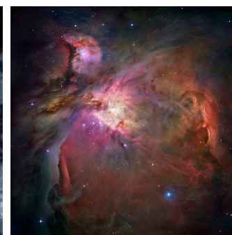
Fig. 8. Nebuloasa Orion
