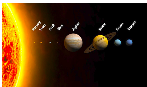
Fig. 1. Planetele Sistemului Solar
